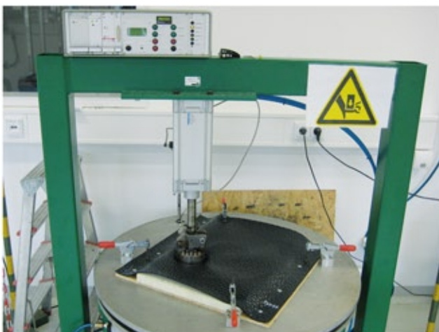
Bild 3: Dauertrittbelastung
