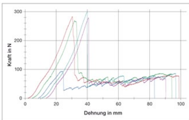
Bild 7: Kraftverlauf Reißfestigkeitsmessungen bei den längs ausgestanzten Schulterstäben
